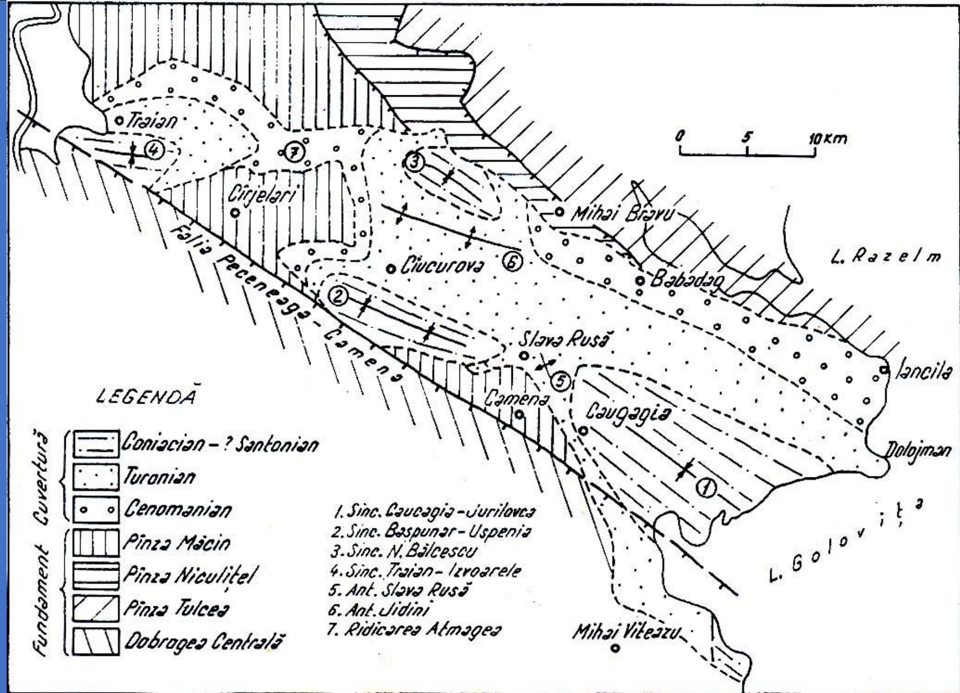
Schița geologică a Platformei Babadag (după O. și El. Mirăuță).
