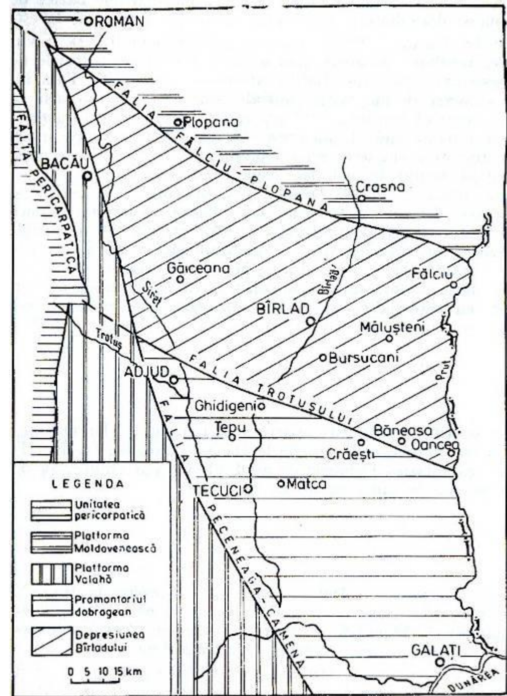
Schița geologică a Depresiunii Bîrladului.
